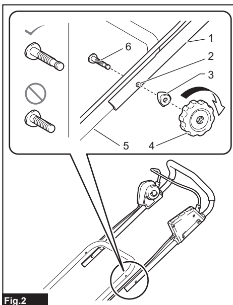
Fig.2 ► 1. Mango superior 2. Orificio 3. Arandela B 4. Tuerca de mano 5. Mango inferior 6. Perno
