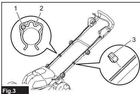
Fig.3 ► 1. Cable 2. Sujetador A 3. Sujetador B
