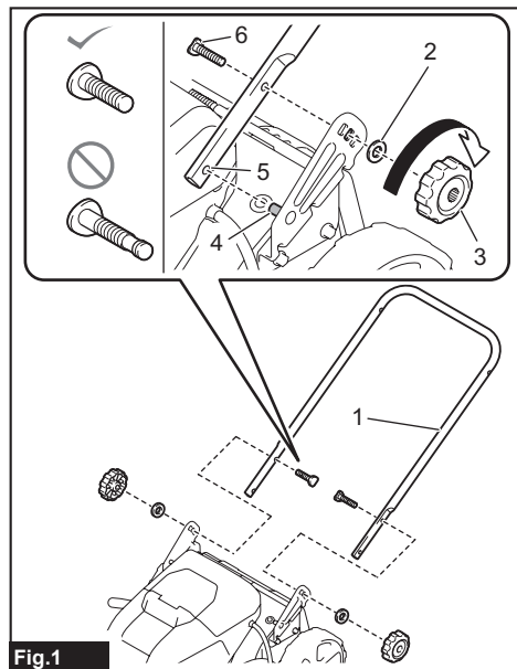
Fig.1 ► 1. Mango inferior 2. Arandela A 3. Tuerca de mano 4. Protuberancia 5. Orificio 6. Perno
